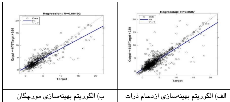
شکل ۳. دقت رگرسیون
